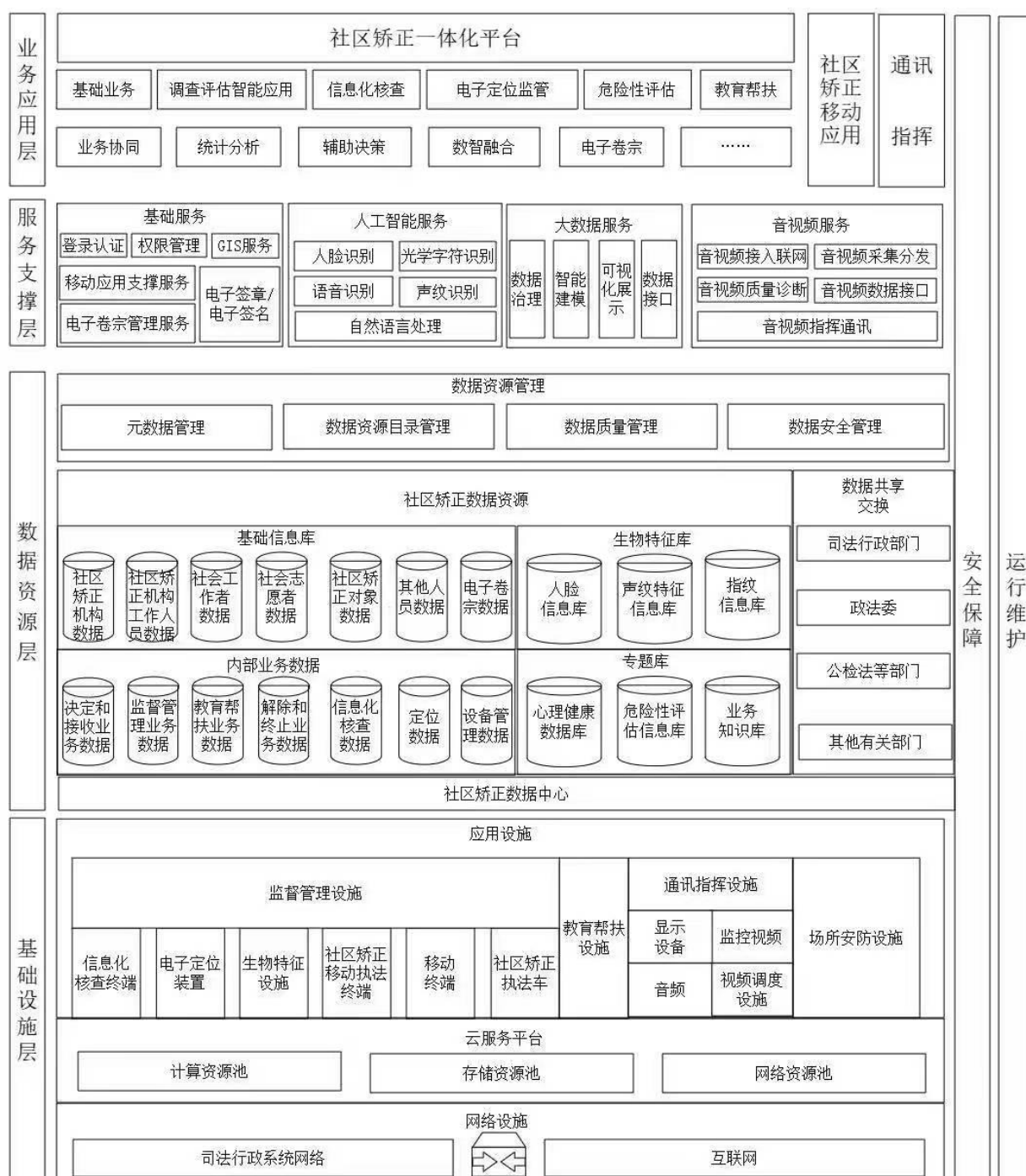
图1 社区矫正信息系统总体架构
