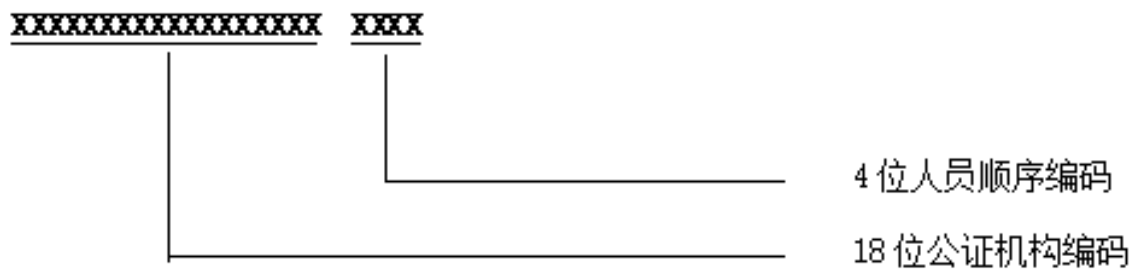
图20 人员编码
