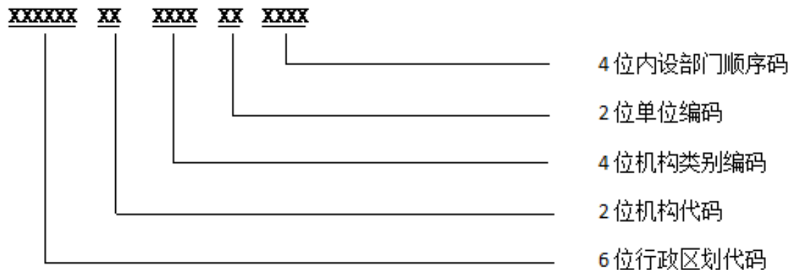
图16 机构编码
